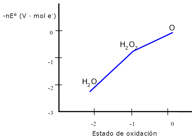
Figura 1. Diagrama de Frost del oxígeno en disolución ácida (pH=0), empleando potenciales estándar de reducción con referencia a E^{\circ} ( H^{+}/H_2 ). En el eje Y se representa -nE^{\circ} , expresado en voltios por mol de electrones (V · mol e - ).
